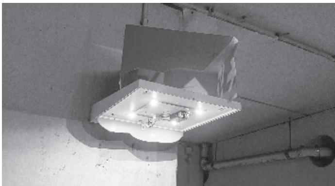
Schäden an der Notausgangsbeleuchtung im P&R-Gebäude
