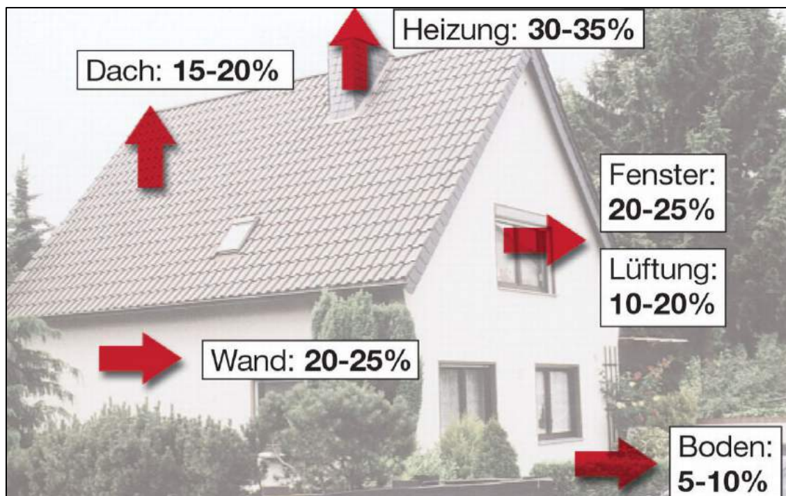
Abbildung 13: Wärmeverluste eines freistehenden Einfamilienhauses, Baujahr 1984 (Quelle: BINE 2003)
